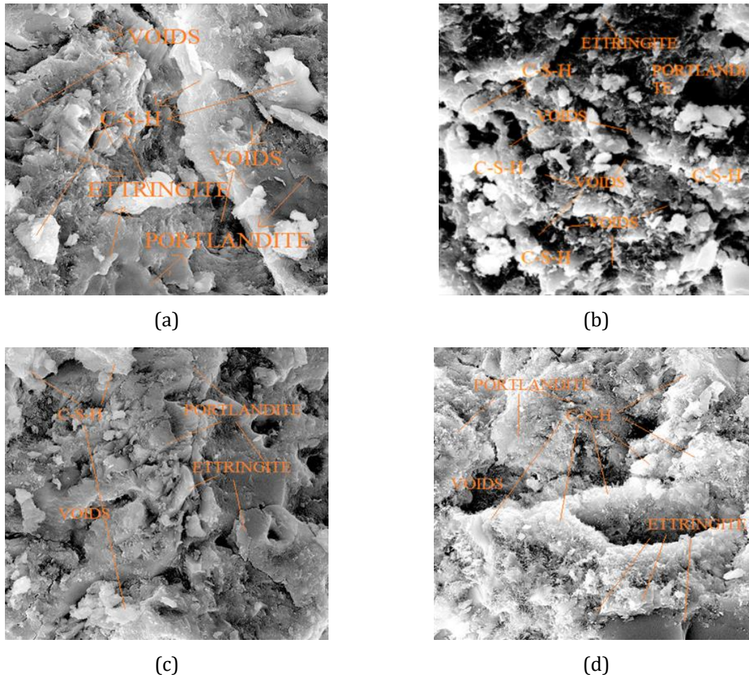
Fig. 19. SEM images (a) A0 mix, (b) A1 mix, (c) B1 mix , and (d) C1 mix
