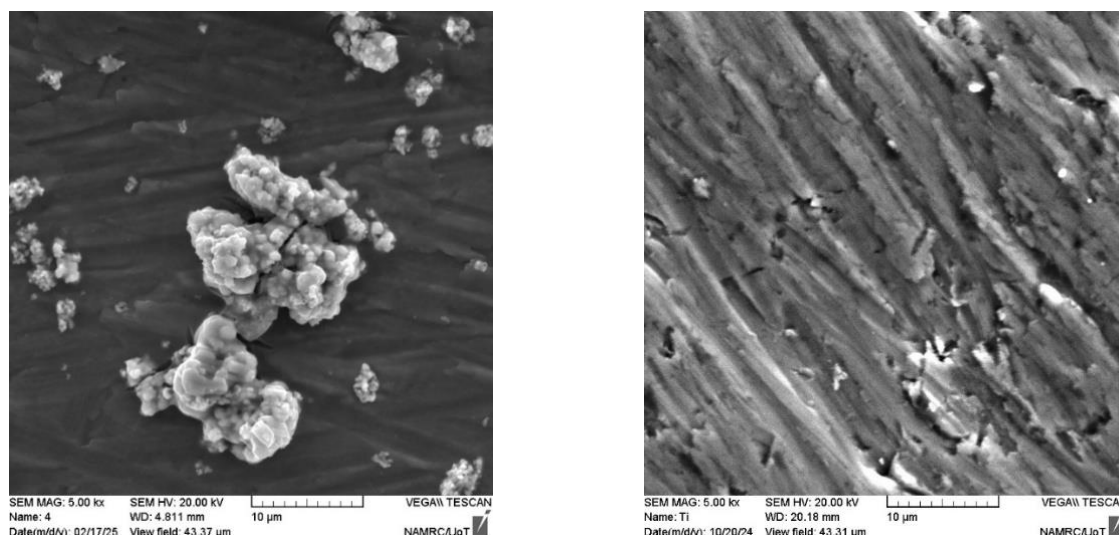
Fig. 2. SEM of Ti – Coated and Pure Ti
